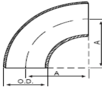
CODO 90° RADIO CORTO
