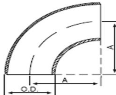
CODO 90° RADIO LARGO
